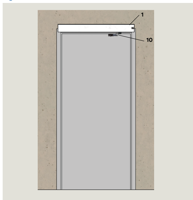
Fig. 8.3.1 ED100/ED250 header
